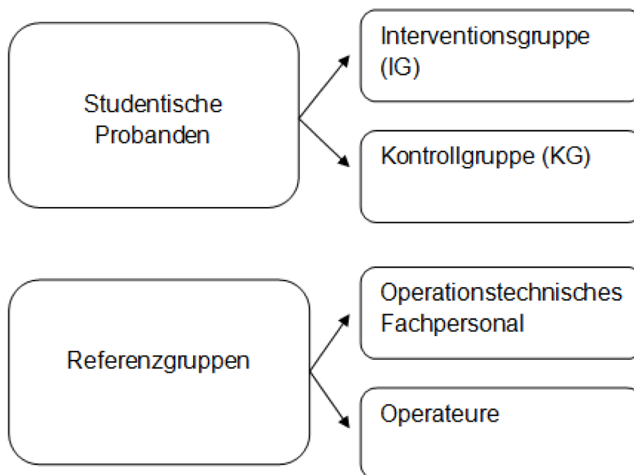
Abbildung 2: Schaubild Kohorteneinteilung
