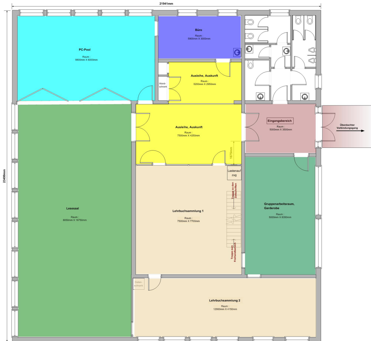
Abbildung 3: FBM-Grundriss Erdgeschoss
